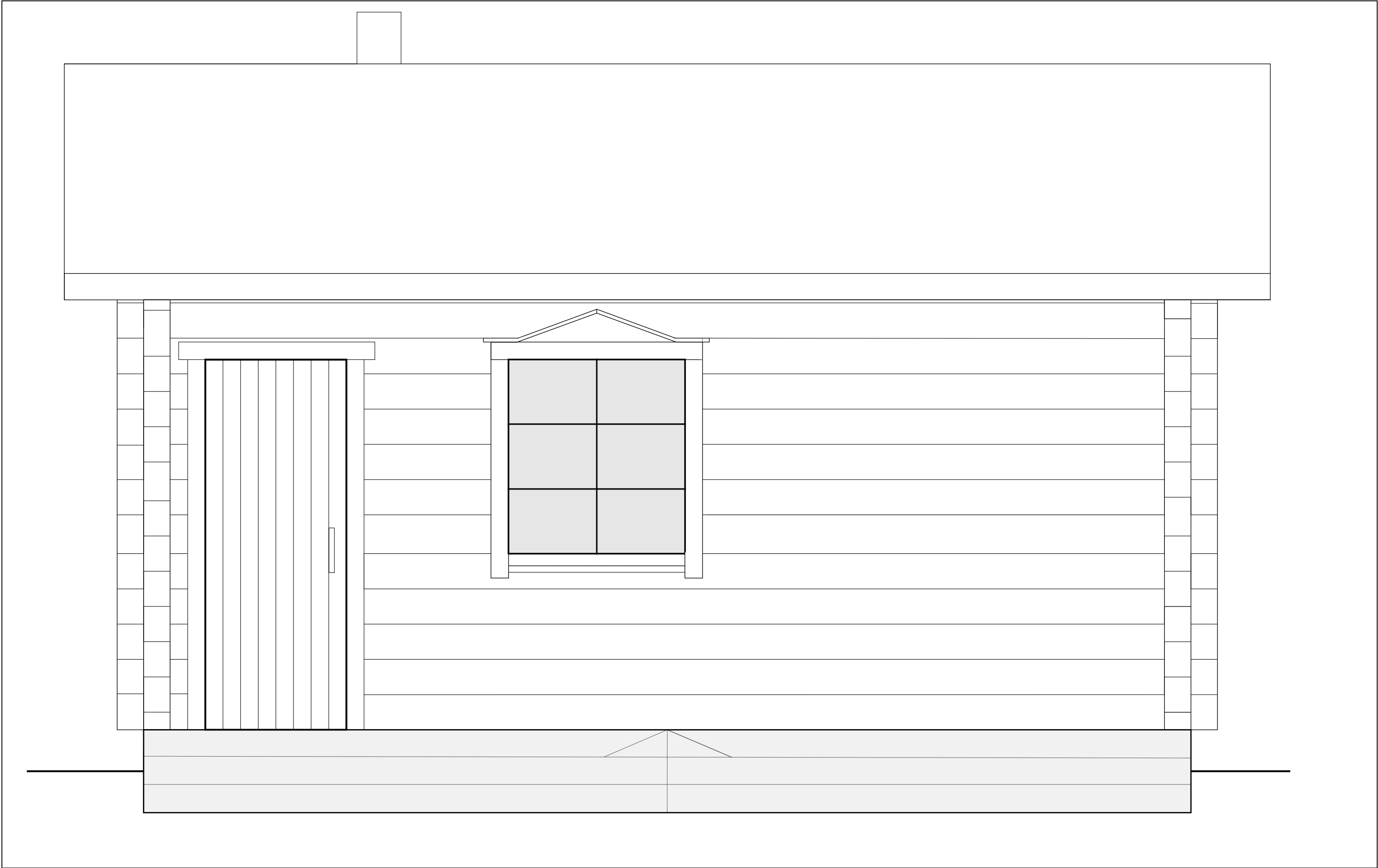
Varaus- / autiotupa julkisivu 1:20
