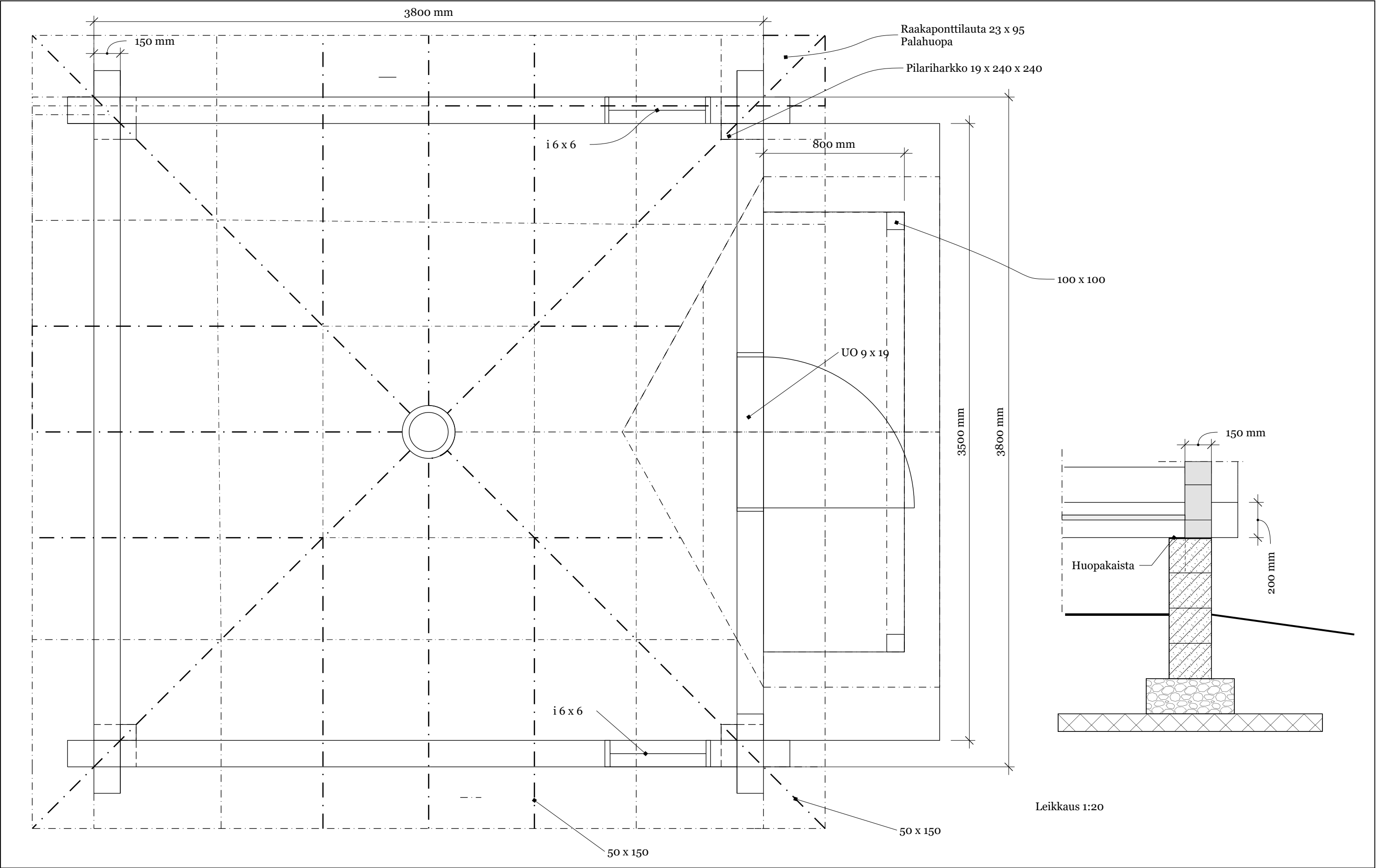
Pohjapiirustus 1:20 Leikkaus 1:20
